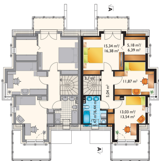
Poddasze 55,93 m 2 / 61,72 m 2
